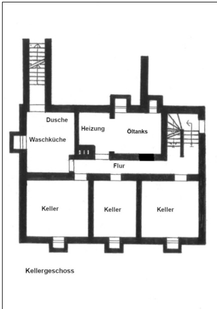
Kellergeschoss
